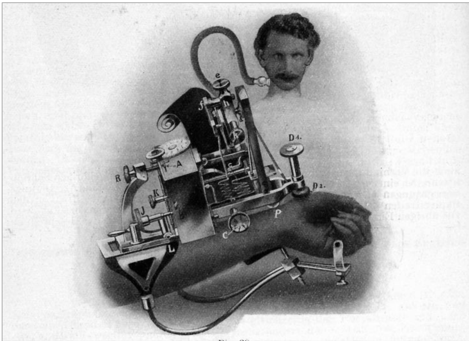
Abbildung 5 Komplexe Technik: Neuer Jacquetscher einfacher Kardiosphygmograph (Sahlbi 1905: 132, Fig. 30)
