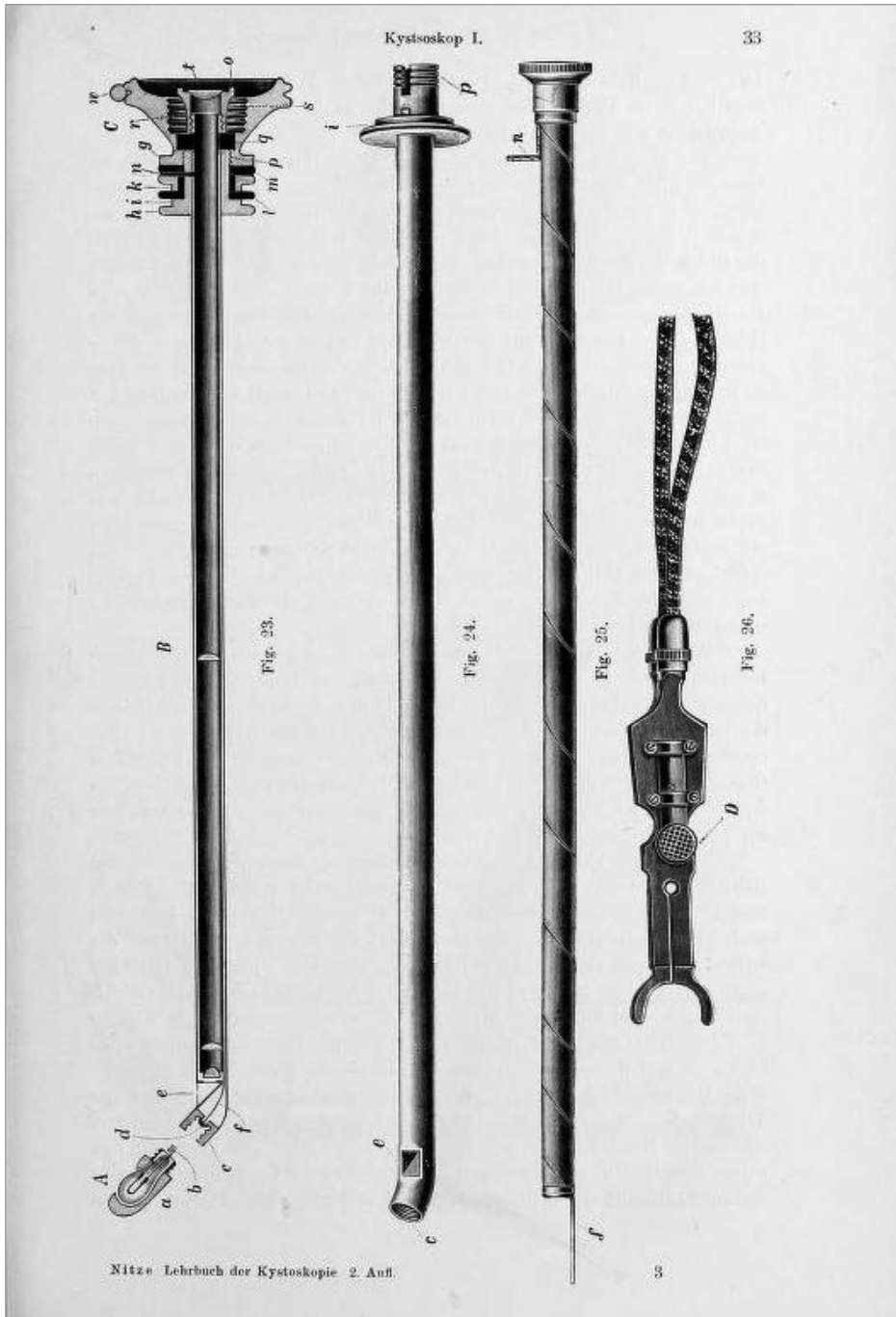
Abbildung 8 Kystoskop I mit Mignonlampe (Nitze 1907: 33)
