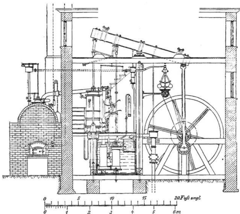
Abbildung 6: Dampfmaschine
