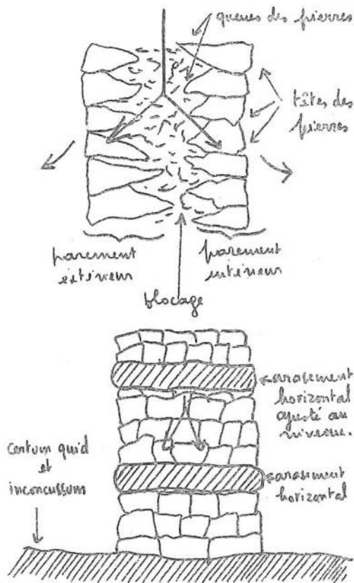
Abbildung 5: Schalenmauerwerk
