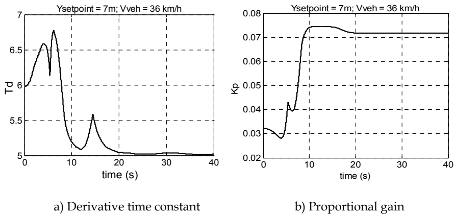
Fig. 15. PD Parameters
