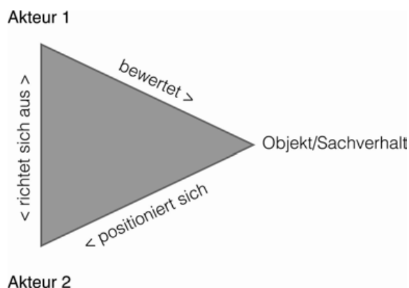
Abb. 2: Stance-Dreieck
