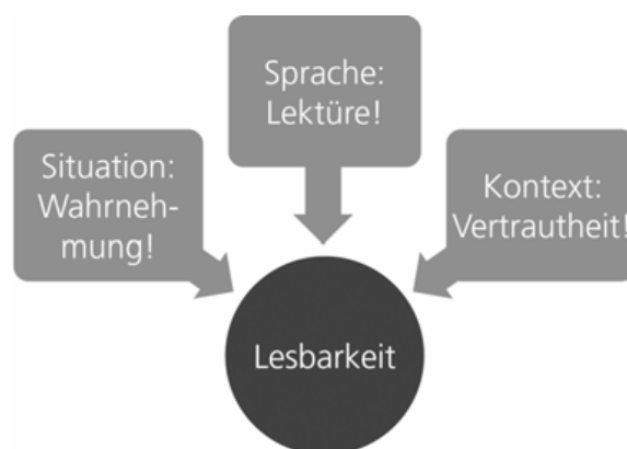
Abb. 4: Lesbarkeitsquellen
