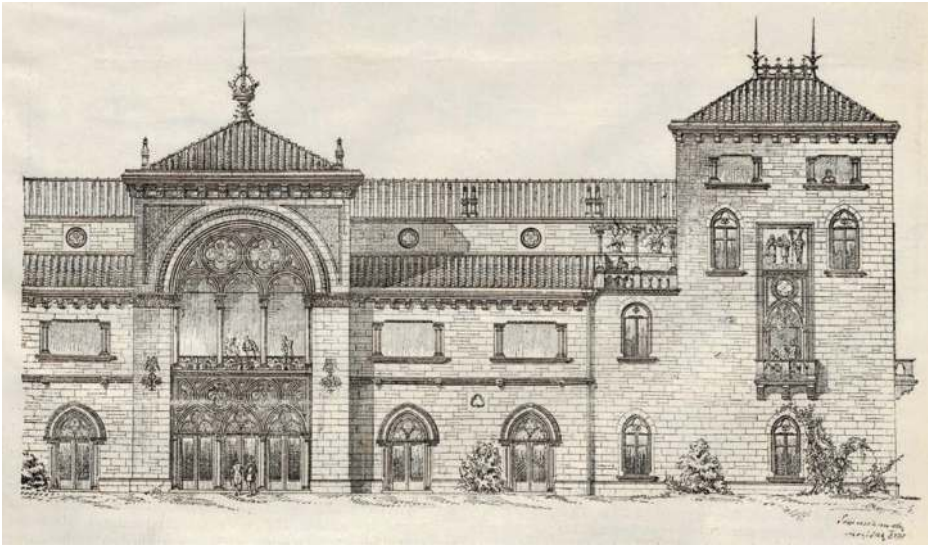
Abb. 6: Franz Xaver Segenschmid, Entwurf für den Kaiserpalast in Lacroma, Detail der Westfassade, um 1864. Der orientalische Salon war im Erdgeschoss im Bereich des risalitartigen Vorbaus als zentraler Mittelsaal und mit direktem Terrassenzugang geplant.
