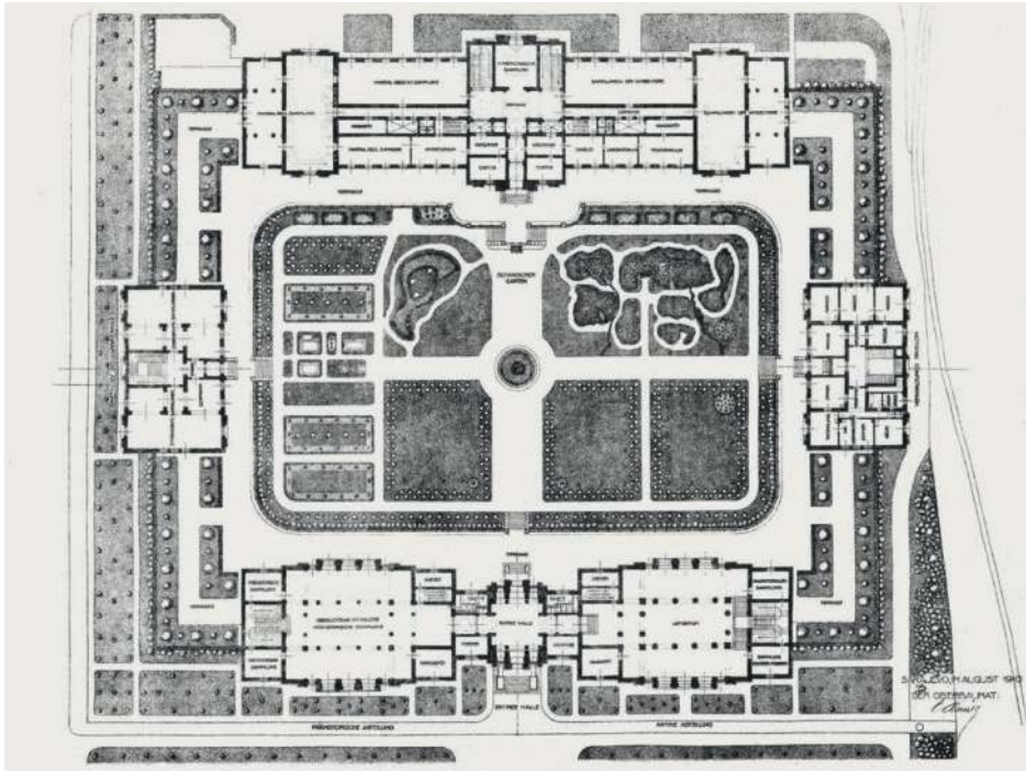
Abb. 1: Sarajevo, Landesmuseum, err. 1909–13, Arch. Karl Pařík, Plan der Gesamtanlage. Quelle: Pařík, Landesmuseum , Taf. 23.
