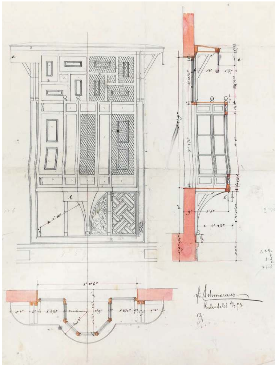
Abb. 2: Franz Schmoranz, Plan für flache maşrabiyya mit Polygonal-Erker im I. Stock des Arabischen Wohnhauses des Ägyptischen Pavillons auf der Wiener Weltausstellung 1873.
