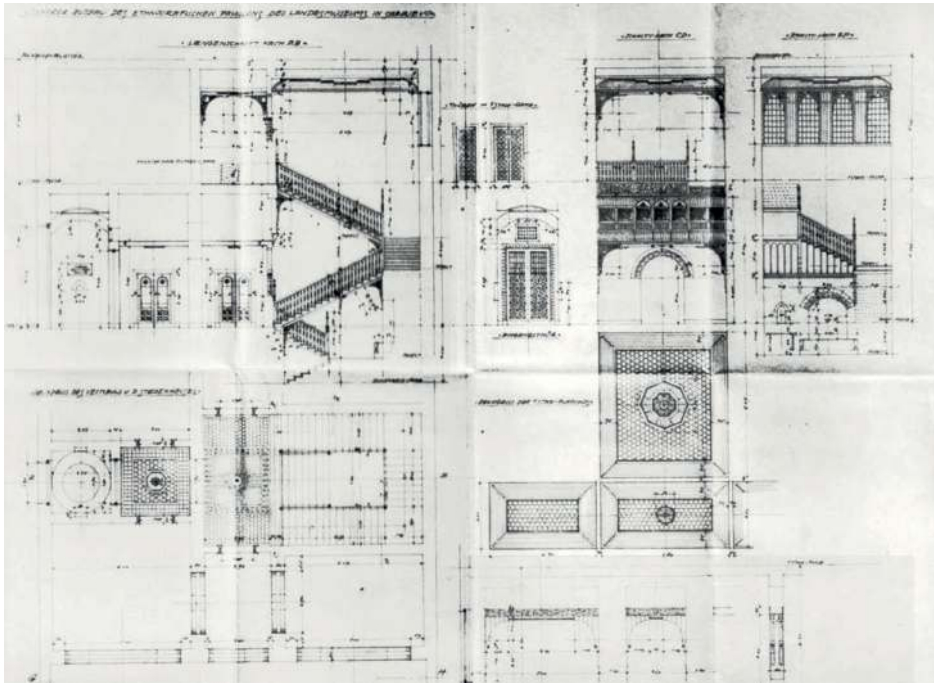
Abb. 9: Projektzeichnung »Innerer Ausbau des Ethnografischen Pavillons des Landesmuseums in Sarajevo« von Josef Pospíšil, 1912 (September).
