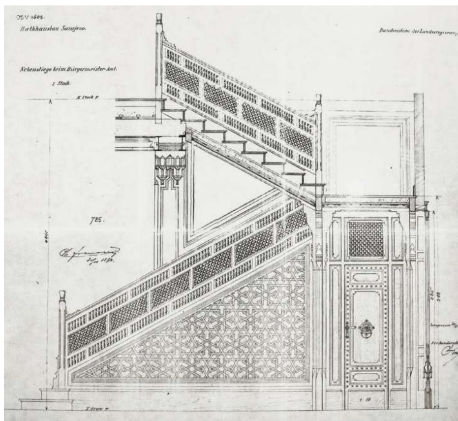
Abb. 10: Zeichnung »Rathausbau Sarajevo. Nebenstiege beim Bürgermeister-Amt. I. Stock« von Arch. Ćiril Iveković, 1894.
