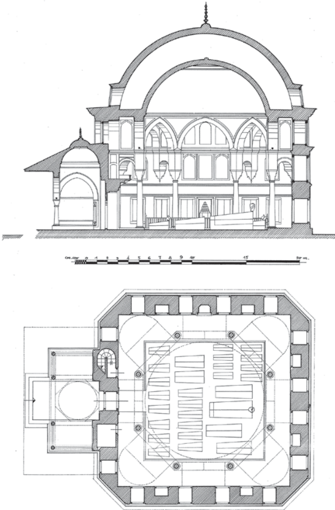
Figure 7.10. Plan and section of the the Mausoleum of Sultan Selim II. From Ali Saim Ülgen, Mimar Sinan Yapıları (Ankara: Türk Tarih Kurumu, 1989).
