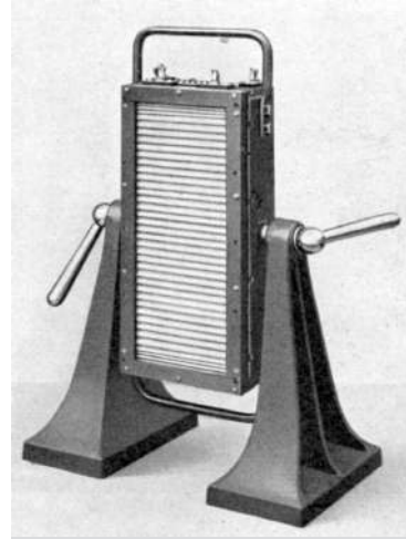
Abb. 100: Der sogenannte „Blatthaller“, ein elektro-dynamischer Lautsprecher von Siemens & Halske, abgebildet in Fritz Fischer u. Hugo Lichte (Hg.): Tonfilm. Aufnahme und Wiedergabe nach dem Klangfilm-Verfahren (System Klangfilm-Tobis) , Leipzig: Hirzel 1931, Abb. 155. Quelle: Österreichische Zentralbibliothek für Physik (Wien), 1755.
