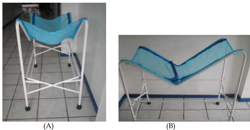
Fig. 9. Bath chair: (A) anterior view; (B) side view.
