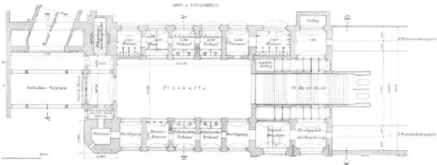
Abbildung 39: Grundriss des Anschlussbahnhofes der Wannseebahn an den Potsdamer Bahnhof.
